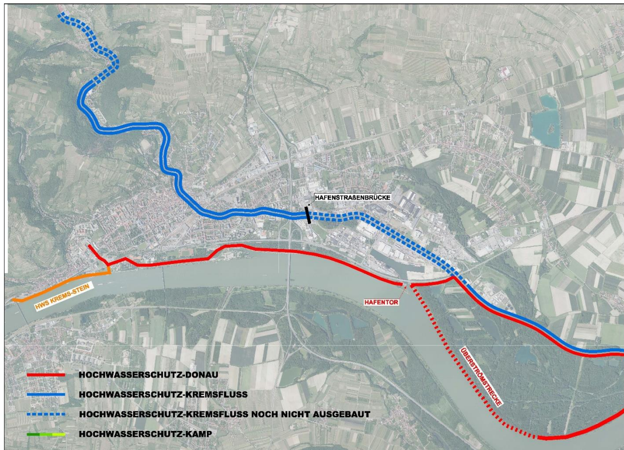
Abbildung 2: Hochwasserschutz in Krems an der Donau
